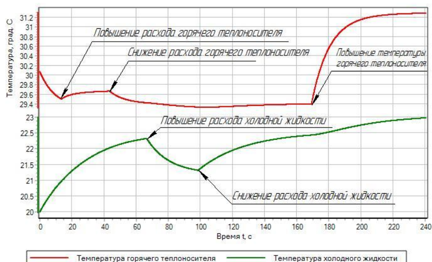
Рис. 3 – Результаты моделирования теплообменного аппарата
