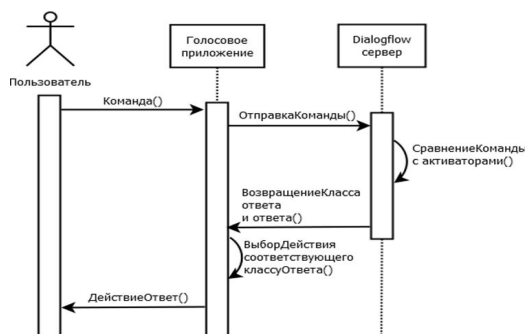
Рисунок 1 - Диаграмма последовательности голосового помощника
